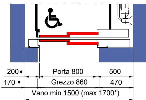
PIANTA VANO CORSA TELAIO PORTE NF (EI120)
